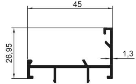
16506 0,385 Kg/Mt
