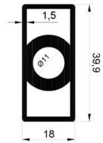
16292 0,874 Kg/Mt
