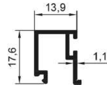
16511 0,176 Kg/Mt
