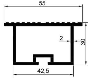
16291 0,945 Kg/Mt
