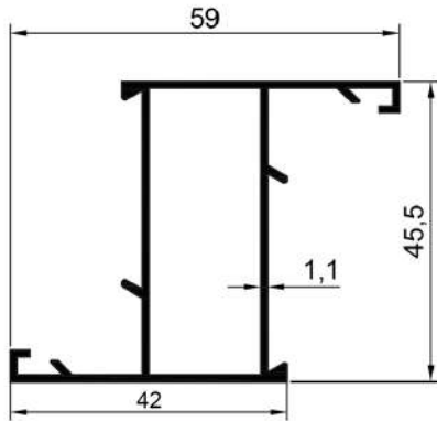
16602 0,568 Kg/Mt
