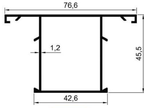
16605 0,708 Kg/Mt
