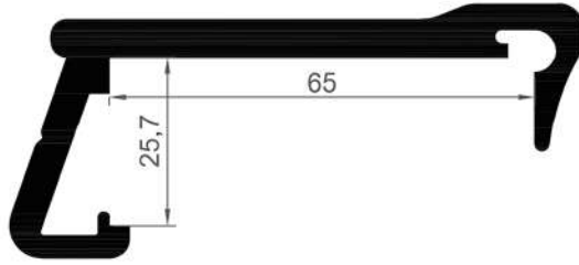
16157 2,032 Kg/Mt
