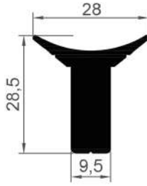
16038 0,775 Kg/Mt
