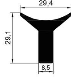
16009 0,750 Kg/Mt
