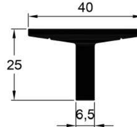
16310 0,777 Kg/Mt
