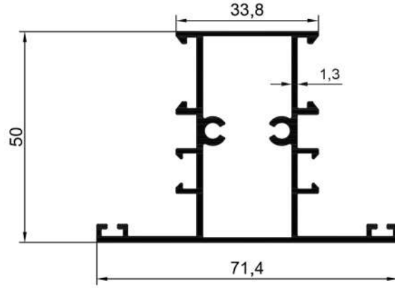
16428 0,965 Kg/Mt
