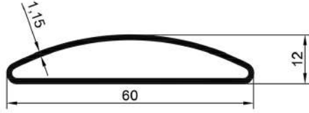
16452 0,390 Kg/Mt
