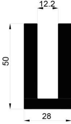
16616 0,591 Kg/Mt
