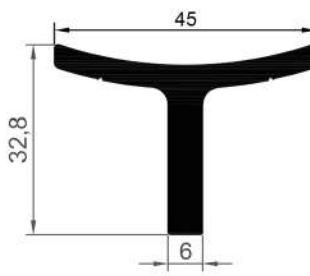
16229 0,908 Kg/Mt
