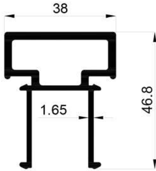
16731 0,972 Kg/Mt
