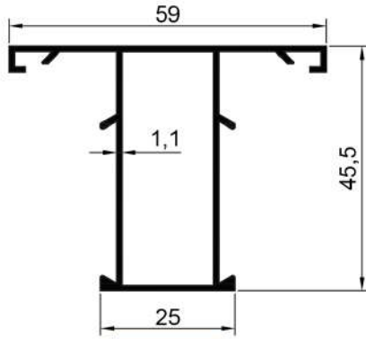
16603 0,568 Kg/Mt
