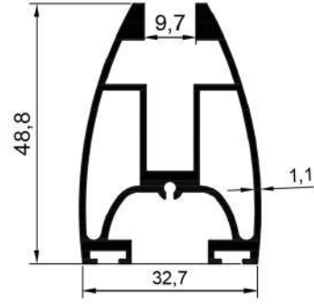
16300 0,830 Kg/Mt
