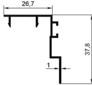
16437 0,255 Kg/Mt
