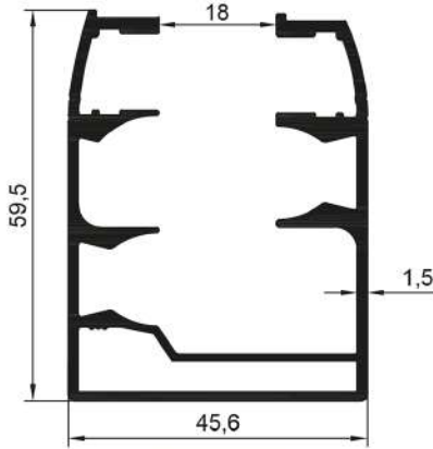
16326 1,230 Kg/Mt
