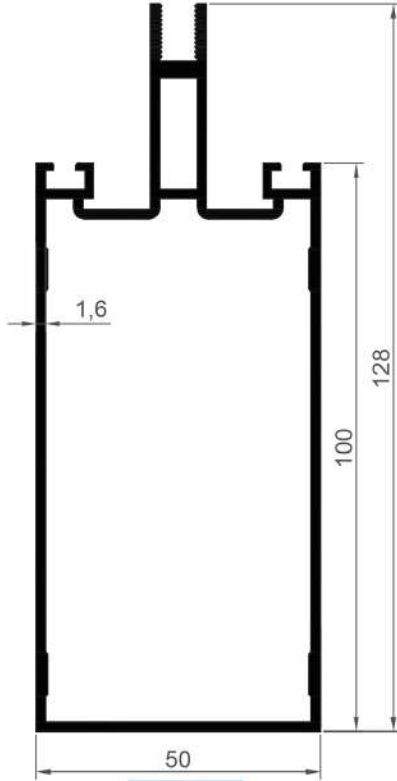
16284 1,774 Kg/Mt
