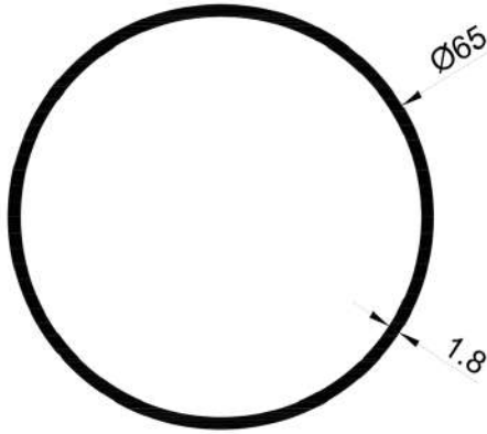
16065 0,910 Kg/Mt
