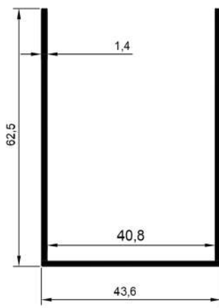
16905 0,610 Kg/Mt
