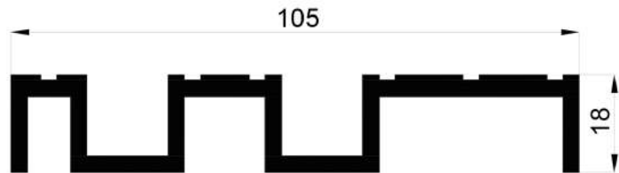
16307 1,685 Kg/Mt
