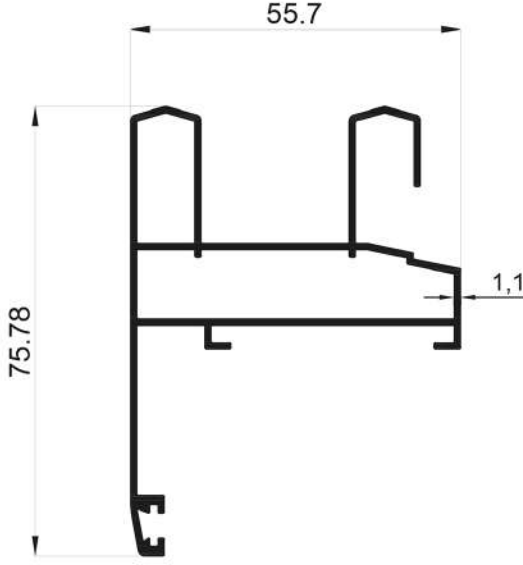
16439 0,926 Kg/Mt
