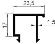
16218 0,272 Kg/Mt
