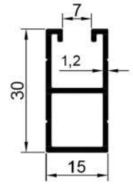
16220 0,304 Kg/Mt
