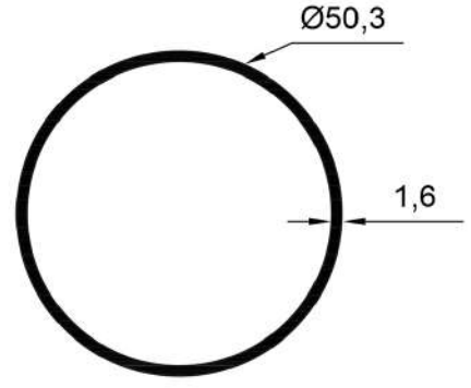
16500 0,705 Kg/Mt
