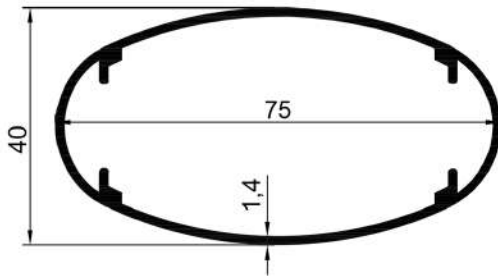
16185 0,812 Kg/Mt
