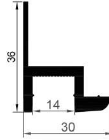
16275 0,555 Kg/Mt
