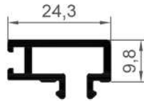
16801 0,271 Kg/Mt
