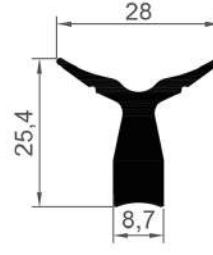
16282 0,533 Kg/Mt
