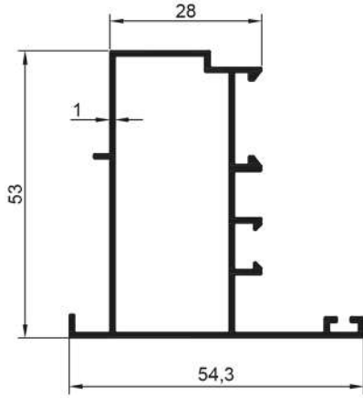
16432 0,610 Kg/Mt
