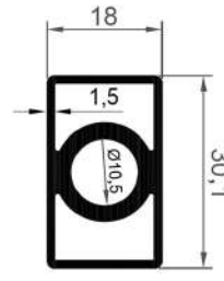
16172 0,580 Kg/Mt
