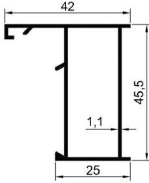
16601 0,504 Kg/Mt
