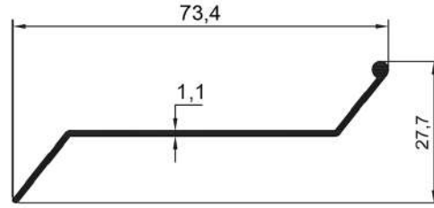
16426 0,285 Kg/Mt
