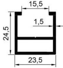
16144 0,391 Kg/Mt
