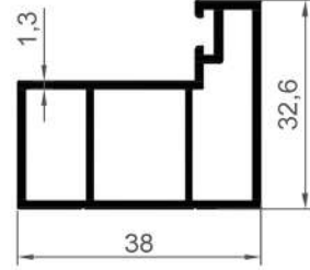
16277 0,593 Kg/Mt
