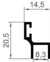
16212 0,158 Kg/Mt
