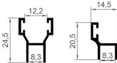
16209 0,226 Kg/Mt
