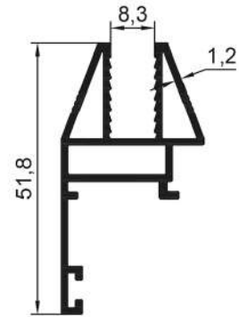
16330 0,575 Kg/Mt
