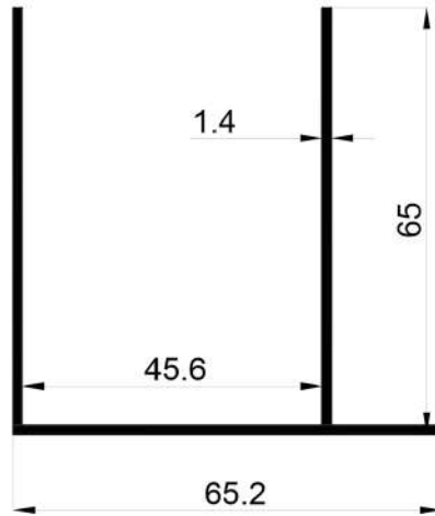
16314 0,740 Kg/Mt
