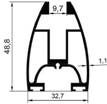
16300 0,830 Kg/Mt
