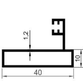
16210 0,437 Kg/Mt
