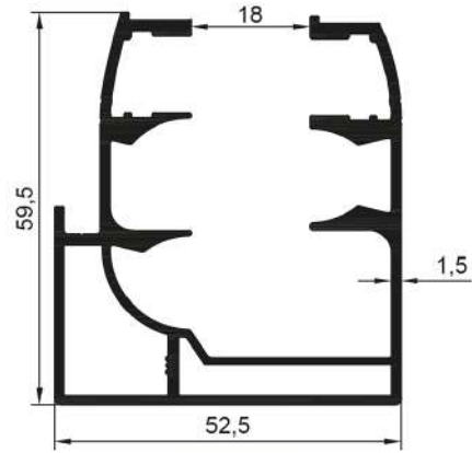
16327 1,348 Kg/Mt
