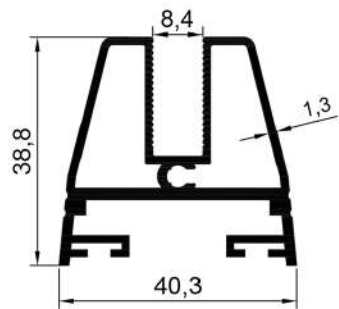
16279 0,901 Kg/Mt
