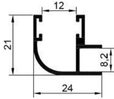
16211 0,260 Kg/Mt
