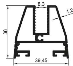
16328 0,829 Kg/Mt
