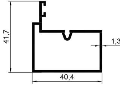
16446 0,580 Kg/Mt
