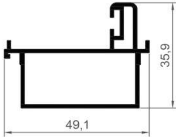
16299 0,596 Kg/Mt
