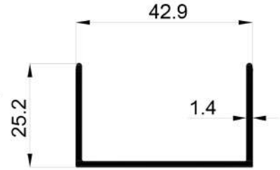
16443 0,355 Kg/Mt
