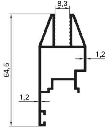
16329 0,680 Kg/Mt
