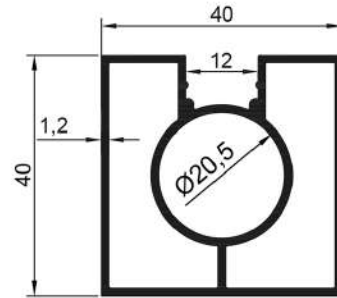
16369 0,816 Kg/Mt
