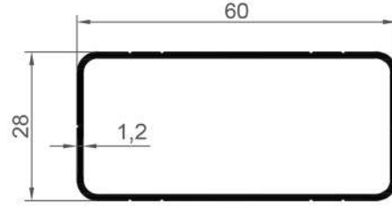
16198 0,536 Kg/Mt
