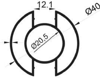
16388 0,596 Kg/Mt
