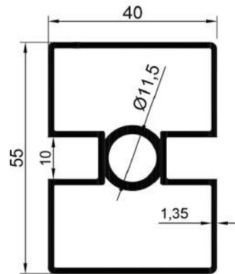
16132 1,041 Kg/Mt
