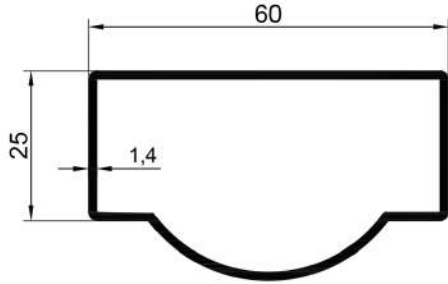
16140 0,640 Kg/Mt
