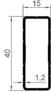
16202 0,342 Kg/Mt
