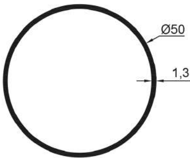
16390 0,538 Kg/Mt
