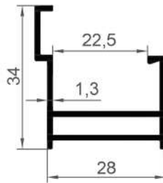
16319 0,409 Kg/Mt
