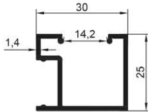
16048 0,795 Kg/Mt
