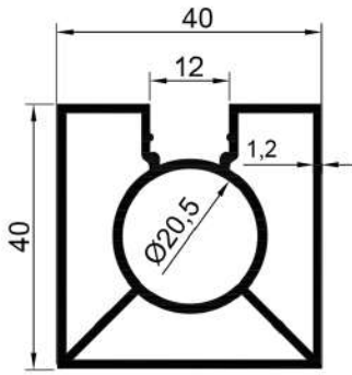
16125 0,950 Kg/Mt
