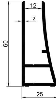
16084 0,870 Kg/Mt
