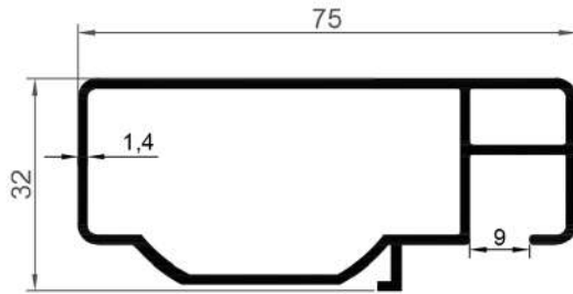
16243 0,886 Kg/Mt
