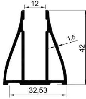
16048 0,795 Kg/Mt
