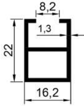
16056 0,250 Kg/Mt
