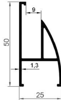
16242 0,509 Kg/Mt
