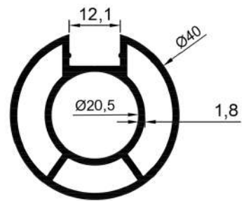
16321 0,970 Kg/Mt
