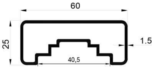
16237 0,749 Kg/Mt
