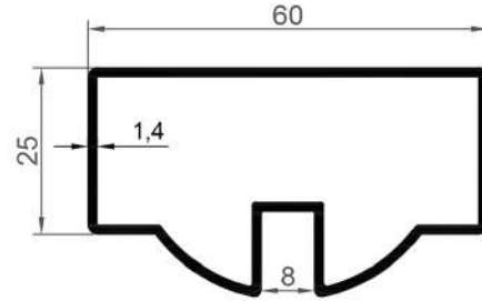
16135 0,736 Kg/Mt
