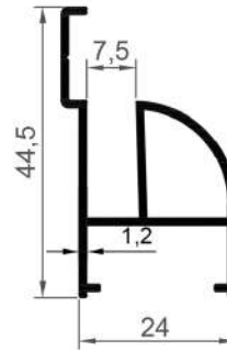
16199 0,423 Kg/Mt
