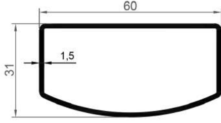
16192 0,660 Kg/Mt
