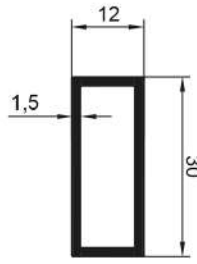
16368 0,320 Kg/Mt
