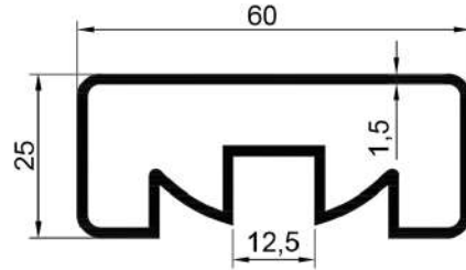
16030 0,823 Kg/Mt
