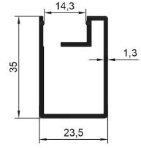
16424 0,435 Kg/Mt
