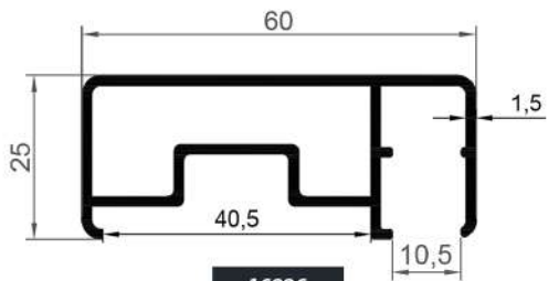
16236 0,782 Kg/Mt
