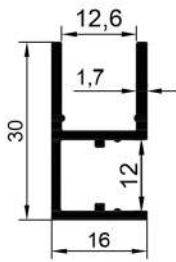
16165 0,330 Kg/Mt
