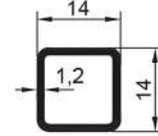
16366 0,165Kg/Mt
