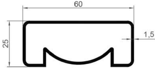
16138 0,733 Kg/Mt
