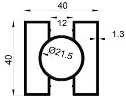
16380 0,860 Kg/Mt
