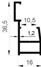
16318 0,308 Kg/Mt
