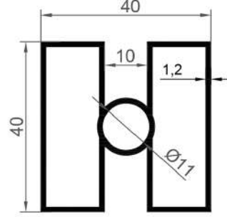
16221 0,755 Kg/Mt
