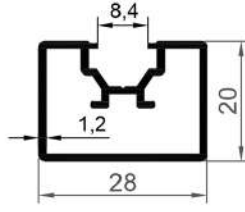
16205 0,363 Kg/Mt
