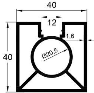
16322 1,100 Kg/Mt
