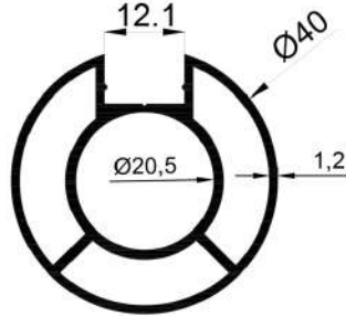
16018 0,720 Kg/Mt
