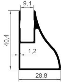
16281 0,417 Kg/Mt
