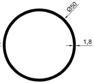
16104 0,735 Kg/Mt
