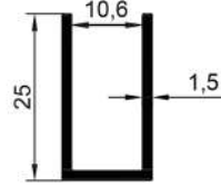
16397 0,255 Kg/Mt
