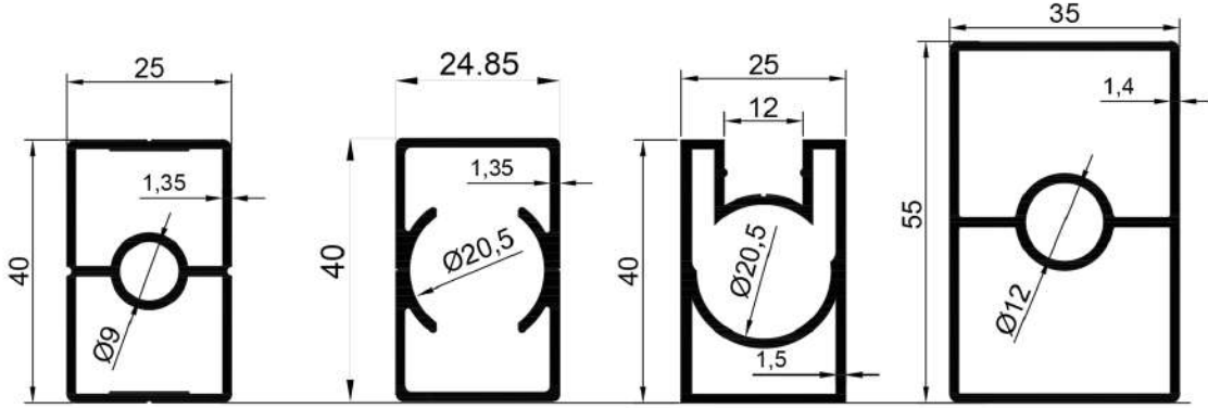
16139 0,627 Kg/Mt
