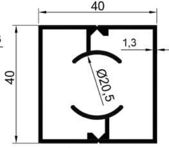
16079 0,785 Kg/Mt
