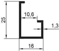
16425 0,205 Kg/Mt
