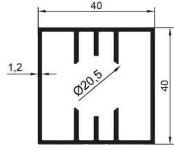
16370 0,730 Kg/Mt
