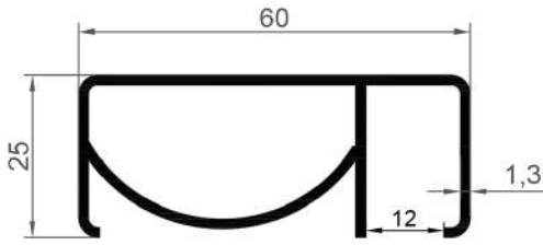
16127 0,675 Kg/Mt
