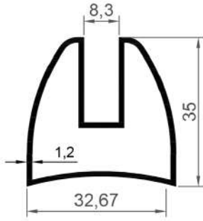
16200 0,531 Kg/Mt
