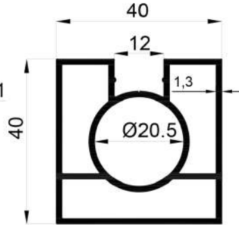
16119 0,920 Kg/Mt
