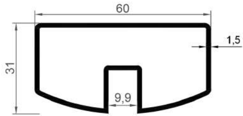
16193 0,776 Kg/Mt
