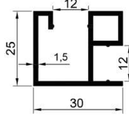
16057 0,470 Kg/Mt
