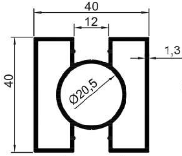
16380 0,851 Kg/Mt
