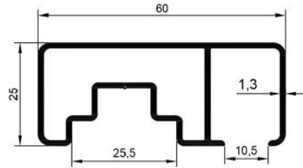
16137 0,700 Kg/Mt
