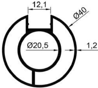
16050 0,690 Kg/Mt
