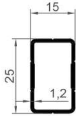
16201 0,246 Kg/Mt
