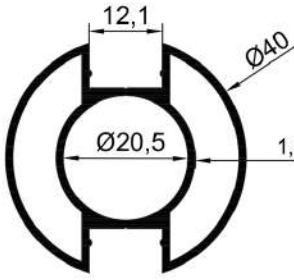
16068 0,690 Kg/Mt
