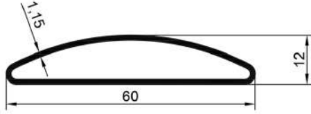
16452 0,390 Kg/Mt
