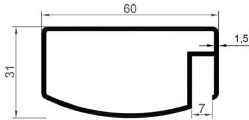
16194 0,732 Kg/Mt
