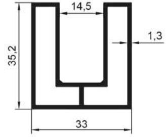
16398 0,675 Kg/Mt
