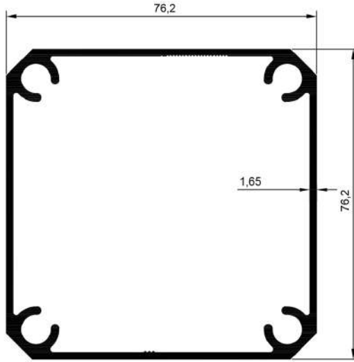
16728 1,707 Kg/Mt
