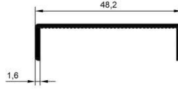
16251 0,257 Kg/Mt
