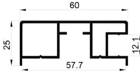
16759 0,711 Kg/Mt
