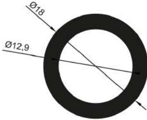
16457 0,345 Kg/Mt
