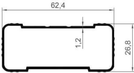
16130 0,535 Kg/Mt
