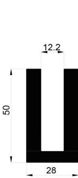
16616 0,591 Kg/Mt
