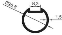
16454 0,275 Kg/Mt
