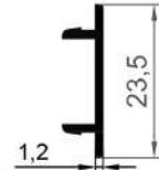
16143 0,110 Kg/Mt
