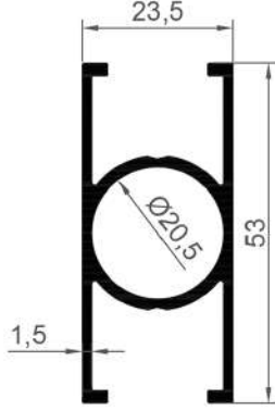
16142 0,739 Kg/Mt
