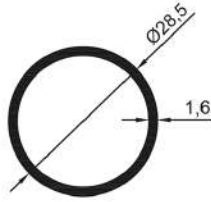
16456 0,380 Kg/Mt
