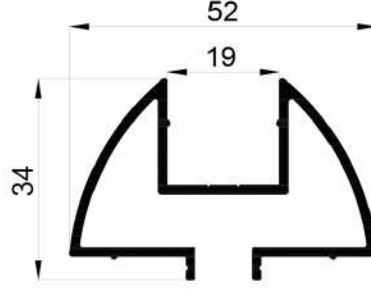
16753 0,693 Kg/Mt
