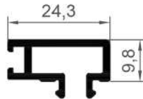
16801 0,271 Kg/Mt
