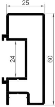
16146 0,830 Kg/Mt
