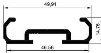
16722 0,546 Kg/Mt
