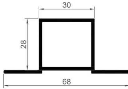
16170 0,691 Kg/Mt
