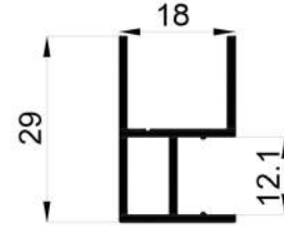
16758 0,294 Kg/Mt
