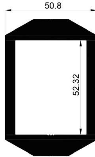
16718 4,085 Kg/Mt
