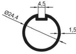
16455 0,325 Kg/Mt
