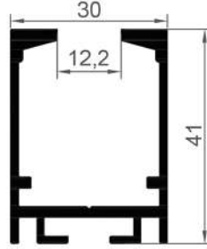
16244 0,717 Kg/Mt
