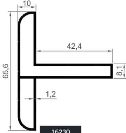
16230 0,750 Kg/Mt
