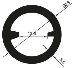
16459 0,795 Kg/Mt
