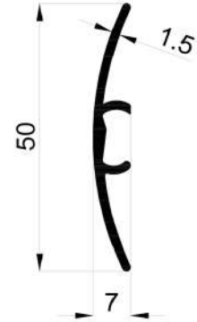
16617 0,270 Kg/Mt
