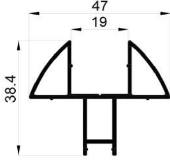
16752 0,555 Kg/Mt
