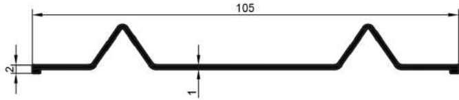
16024 0,394 Kg/Mt
