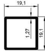
16733 0,247 Kg/Mt
