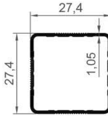
16128 0,294 Kg/Mt
