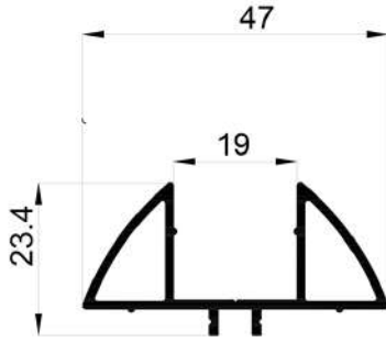
16754 0,455 Kg/Mt
