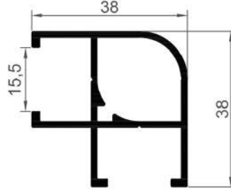
16145 0,650 Kg/Mt
