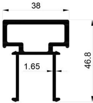
16731 0,972 Kg/Mt
