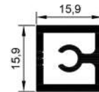
16721 0,324 Kg/Mt
