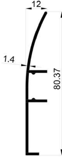
16618 0,425 Kg/Mt
