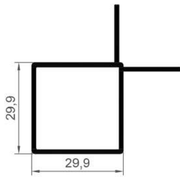
16169 0,572 Kg/Mt
