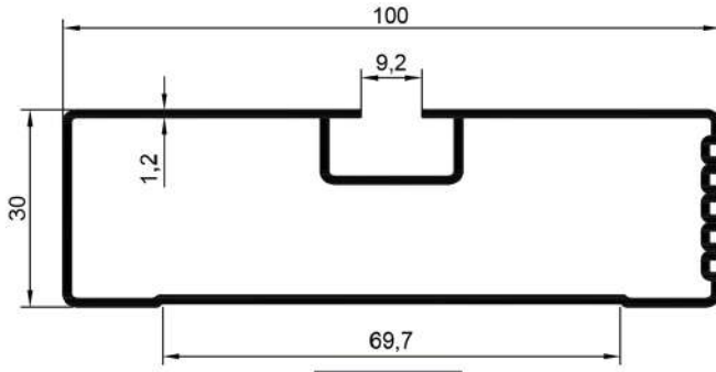
16034 0,965 Kg/Mt
