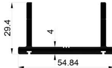
16725 0,983 Kg/Mt
