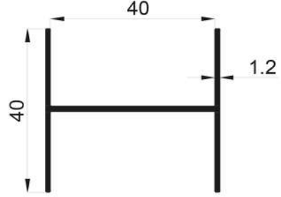
16356 0,395 Kg/Mt
