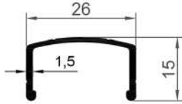
16177 0,175 Kg/Mt
