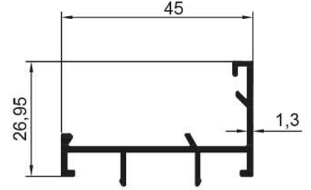
16506 0,385 Kg/Mt
