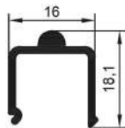
16515 0,175 Kg/Mt
