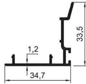
16514 0,280 Kg/Mt
