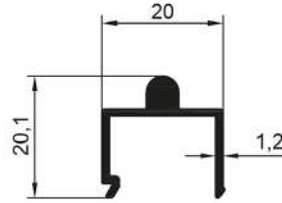
16507 0,385 Kg/Mt
