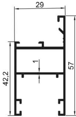
16513 0,530 Kg/Mt
