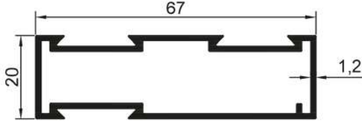
16510 0,692 Kg/Mt
