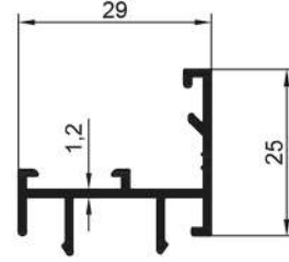
16512 0,300 Kg/Mt
