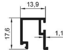
16511 0,176 Kg/Mt
