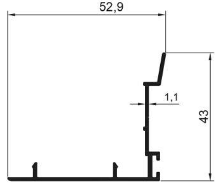
16509 0,350 Kg/Mt
